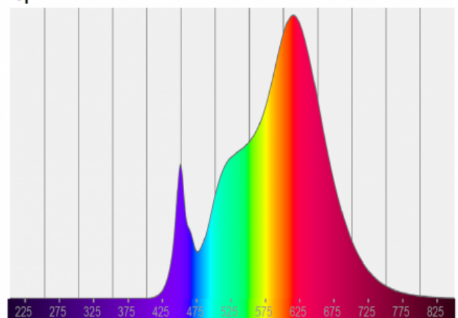
Spectra
